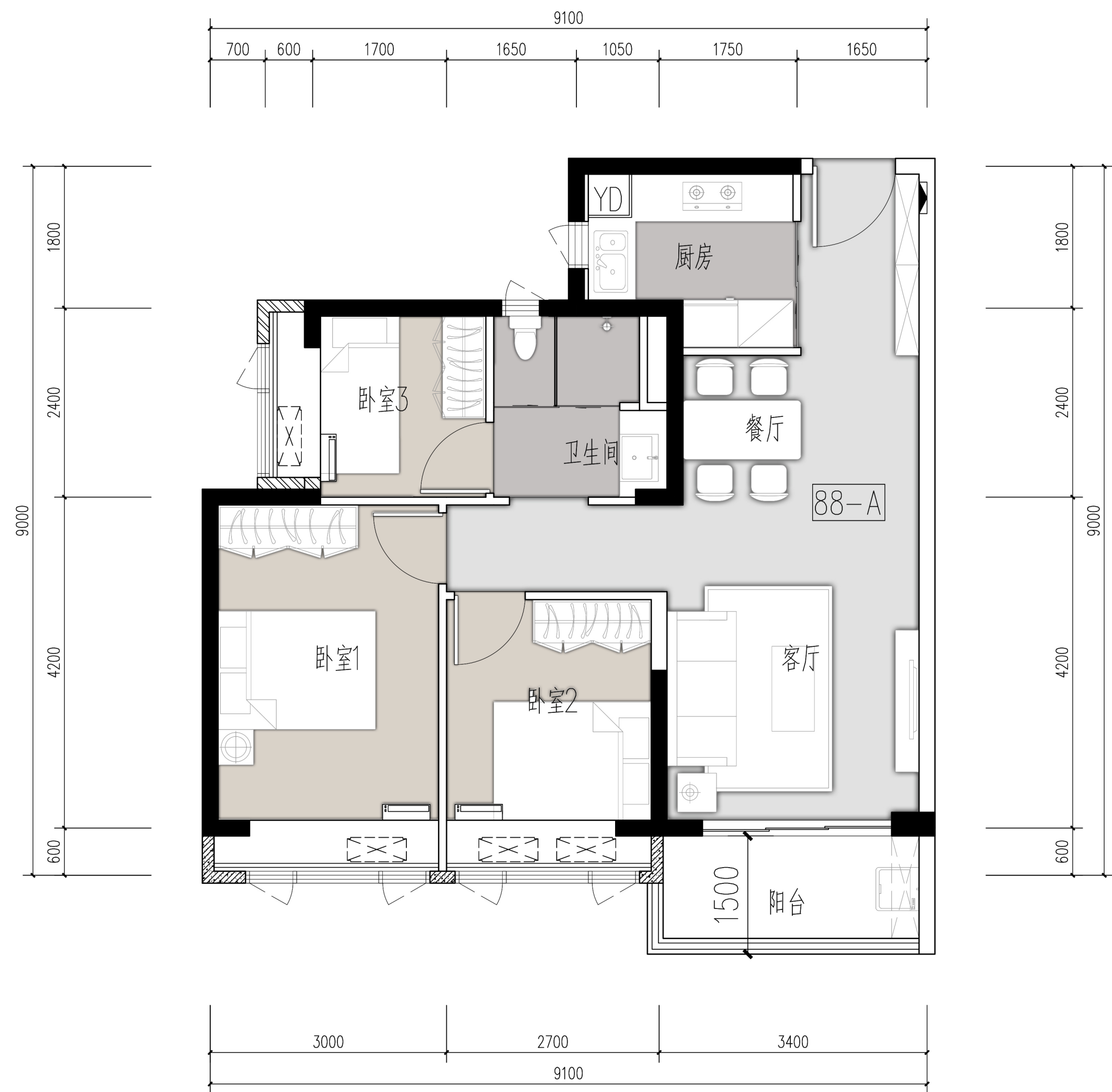
88A户型平面图
