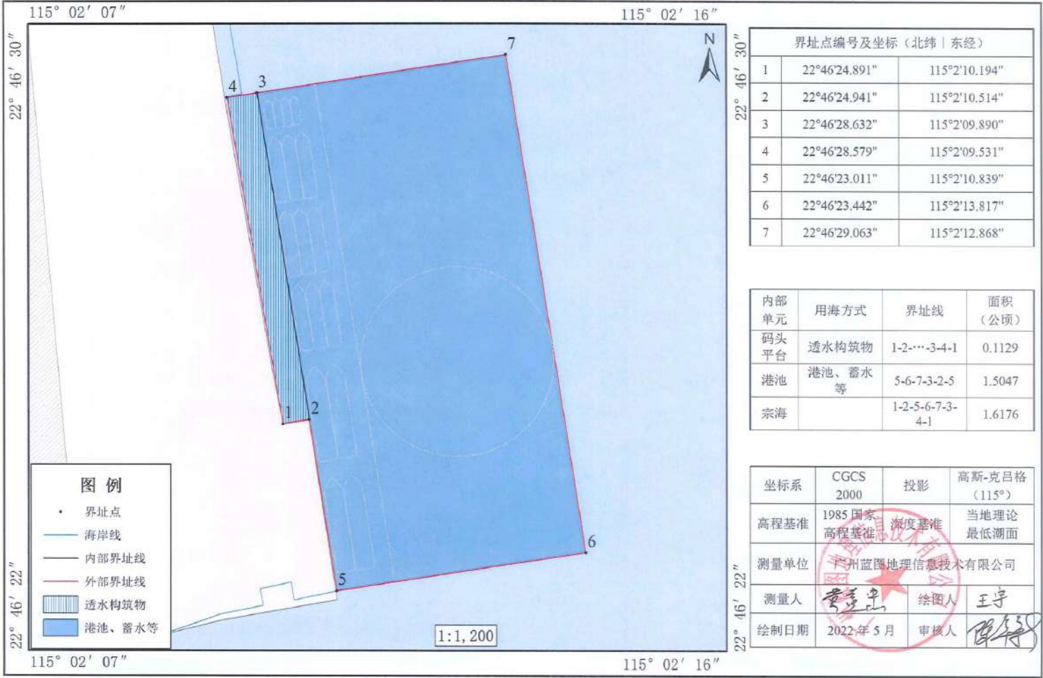
小漠渔港升级改造工程宗海界址图
