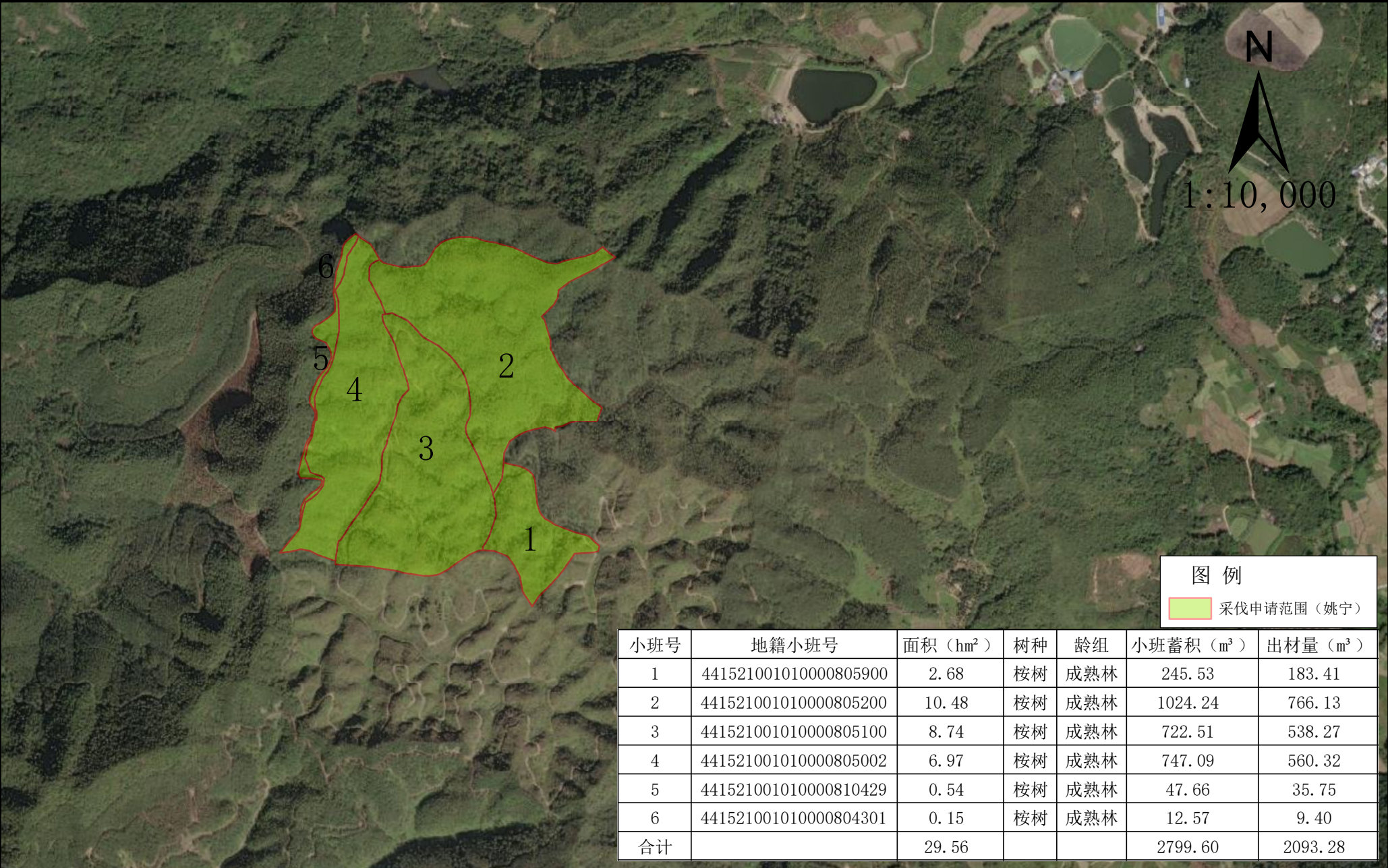
深汕特别合作区赤石街道（镇）大安村委胡安村罗畲林地（姚宁）桉树林采伐作业设计图
